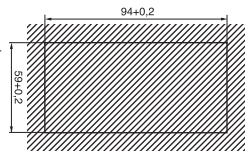
Foratura pannello con uso della mascherina A70R Cut out with use of A70R frame
