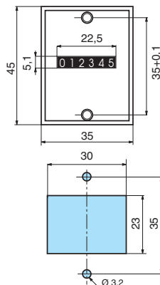
Fissaggio dal fronte Front fixing
